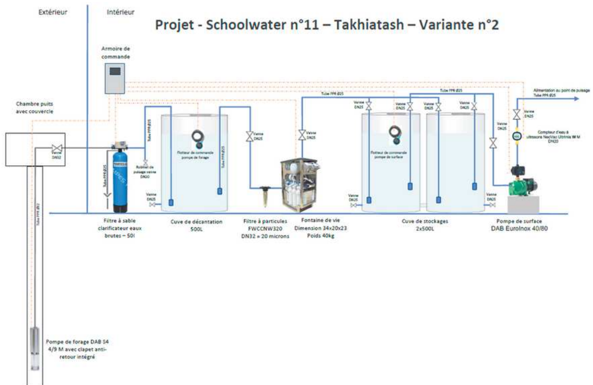
Lavage des mains avec le dispositif The Drop® et schéma de principe de l'installation de traitement d'eau
